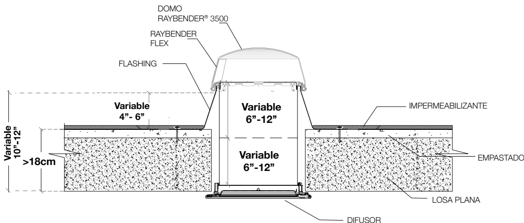
CORTE-SOLATUBE INSTALADO
